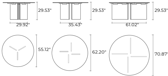
STRUTTURA DV-GLASS® DV-GLASS® STRUCTURE
