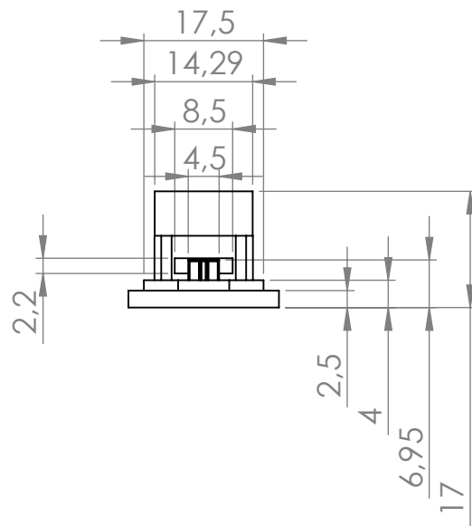
SEZIONE A-A
