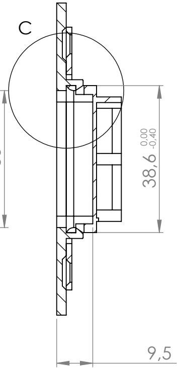
SEZIONE A-A
